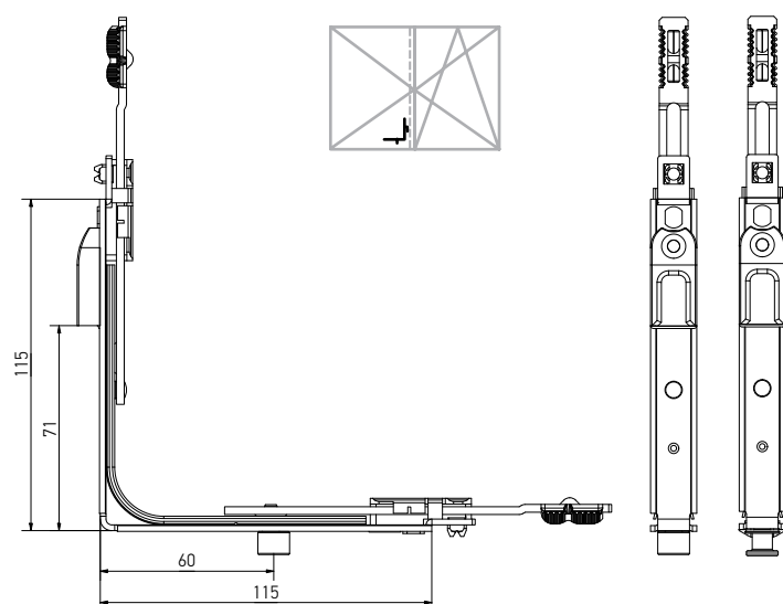
Угловая передача для штульповой створки, 1 ML, 115×115, нижняя
