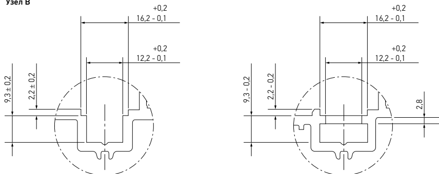
Узел В
