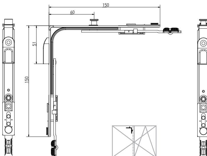
Угловая передача для штульповой створки, 1 MR, 150×150, нижняя
