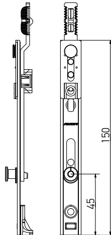
Поворотный шпингалет 90° (нижний), 1 MR
