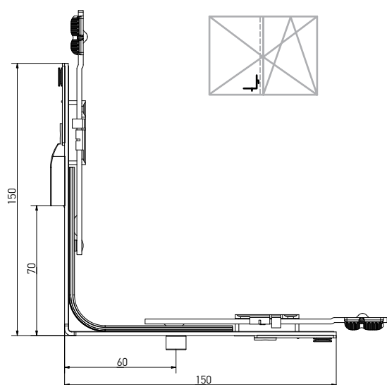
Угловая передача для штульповой створки, 1 ML, 150×150, нижняя
