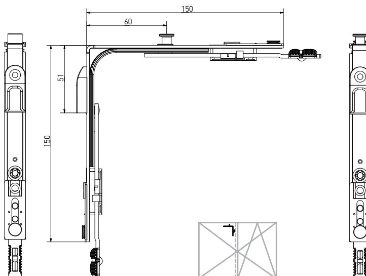
Угловая передача для шпательной створки, 1 MR, 150×150, нижняя
